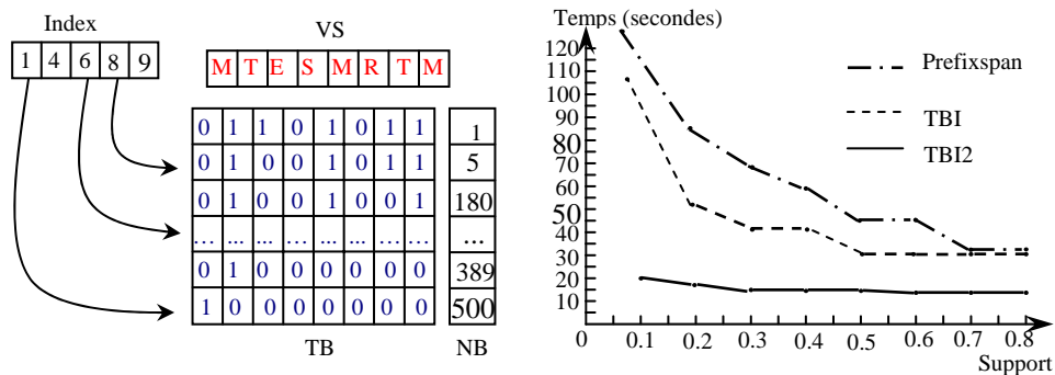
Fig. 1. Structure de données et performance pour 500000 séquences
